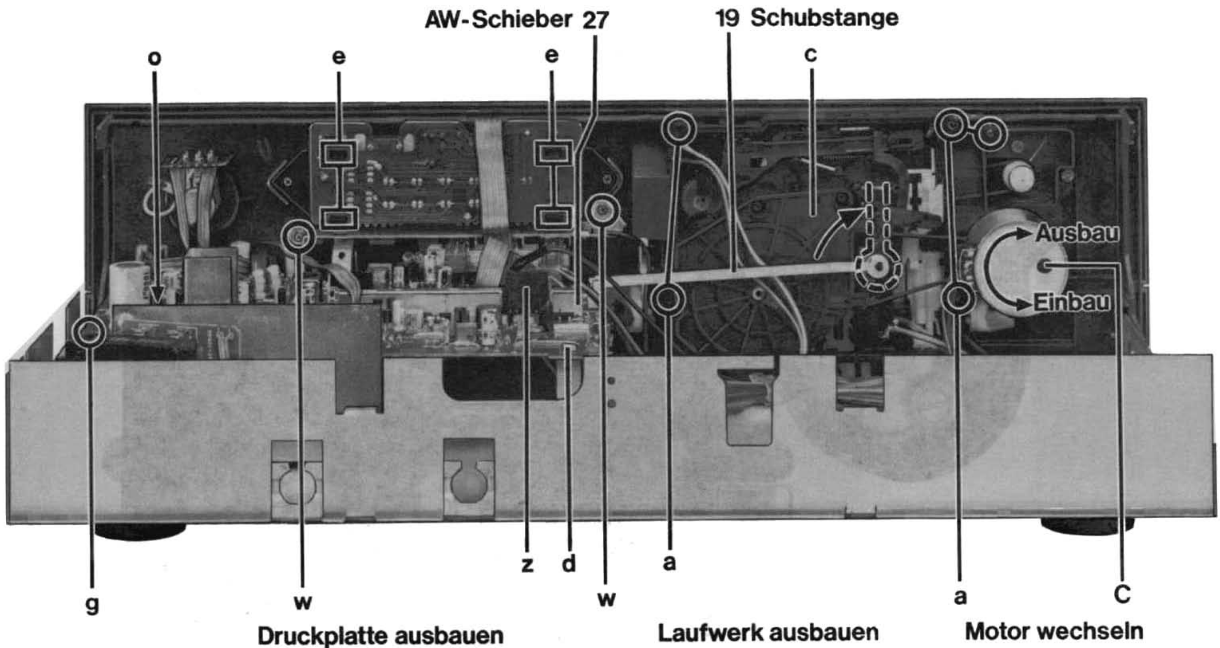
Abb. 2 Innenansicht
